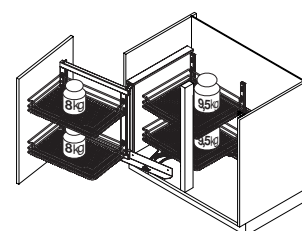
Otočno-výsuvné kovanie pre roh. skrinku WACO, druh koša Saphir, ľavé
