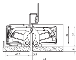
Montáž na oceľovú zárubňu
