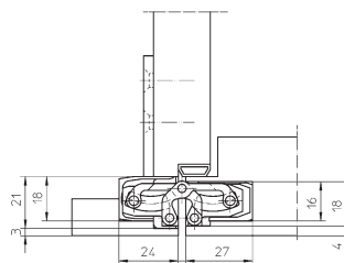
Montáž na obložkovú zárubňu
