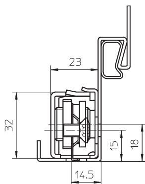
bezfalcový
