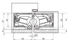
Montáž na rámovú zárubňu
