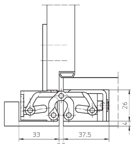
Montáž na obložkovú zárubňu
