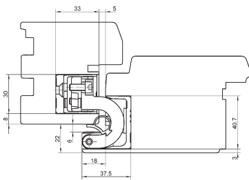
presah 22 mm
