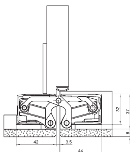
Montáž na obložkovú zárubňu
