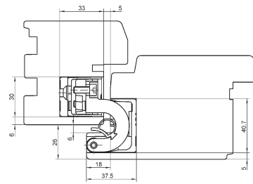
presah 26 mm
