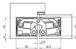
Montáž na rámovú zárubňu
