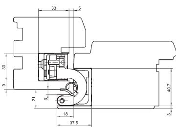
presah 21 mm
