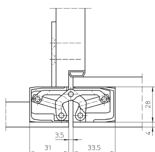
Montáž na obložkovú zárubňu
