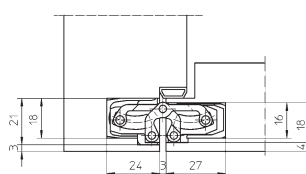
Montáž na rámovú zárubňu
