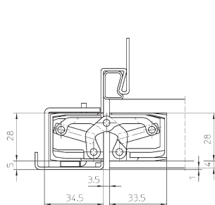
Montáž na oceľovú zárubňu
