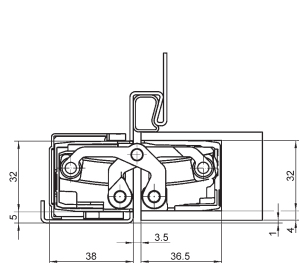
Montáž na oceľovú zárubňu
