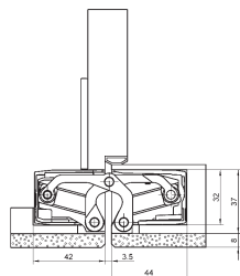
Montáž na obložkovú zárubňu
