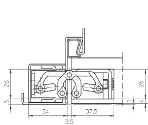
Montáž na oceľovú zárubňu
