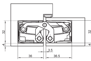
Montáž na rámovú zárubňu
