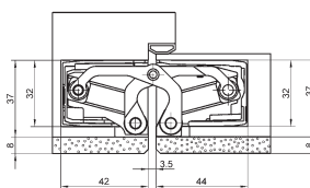
Montáž na rámovú zárubňu
