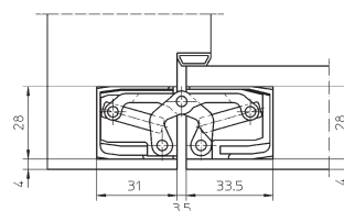
Montáž na rámovú zárubňu
