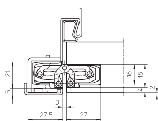
Montáž na oceľovú zárubňu
