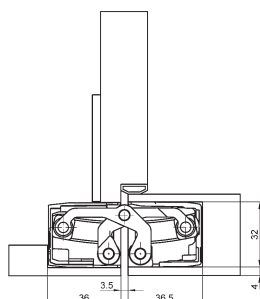
Montáž na obložkovú zárubňu
