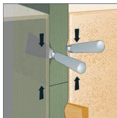
obrázok 2: tupý spoj pri masívnej konštrukcii
